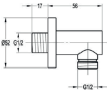
FA4341CP-0: Salida de Agua
